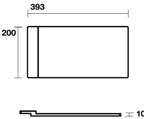
7815 Pianetto per lavabo Kanaal cm 100/120 (5743-5742) Shelf for Kanaal washbasin cm 100/120 (5743-5742)
