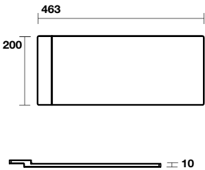
7816 Pianetto per lavabo Kanaal cm 80 (5741) Shelf for Kanaal washbasin cm 80 (5741)
