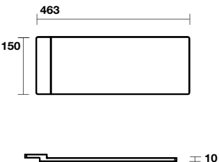
7814 Pianetto per lavabo Kanaal cm 60 (5740) Shelf for Kanaal washbasin cm 60 (5740)
