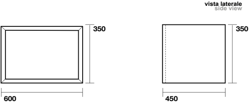
9150 Mobile sospeso cm 60 con vano a giorno Wall hung cabinet cm 60 with open space
