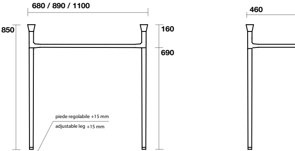
9277-76-75 Struttura a terra per lavabo cm 120-100-80 Steel free standing for washbasin cm 120-100-80
