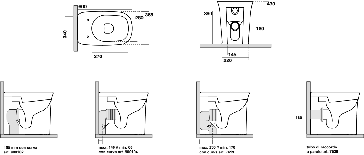
5618 Vaso Btw cm 60 Btw Wc pan cm 60
