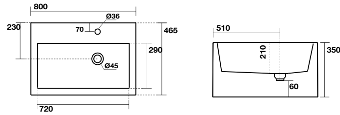
5741 KANAAL lavabo sospeso/appoggio cm 80 KANAAL wall hung or counter top washbasin cm 80
