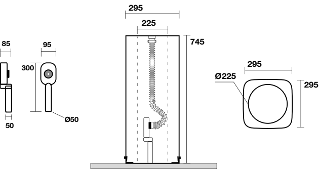
5575 OKE colonna scarico a suolo per Art. 5541 OKE pedestal floor drain for Art. 5541
