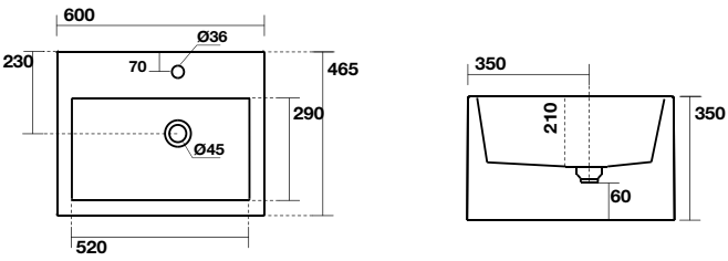
5740 KANAAL lavabo sospeso/appoggio cm 60 KANAAL wall hung or counter top washbasin cm 60
